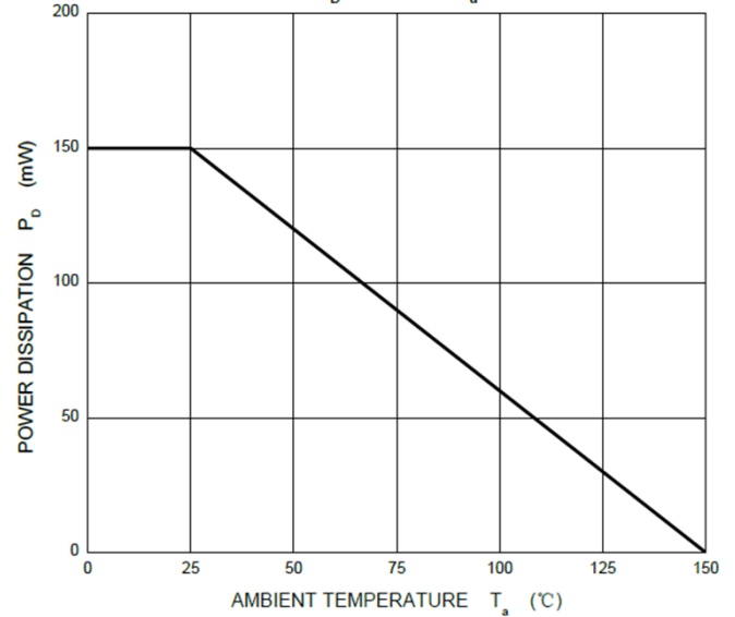
P_D — T_a
