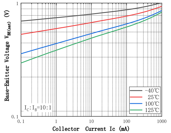
Fig.4 - Base-Emmitter Voltage
